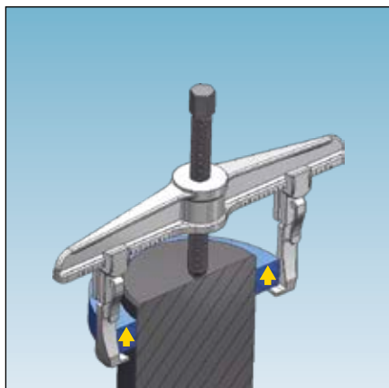
Vnější stahovák HAZET ve standardním provedení
