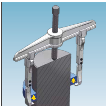
Vnější stahovák HAZET s dlouhým stahovacím hákem
