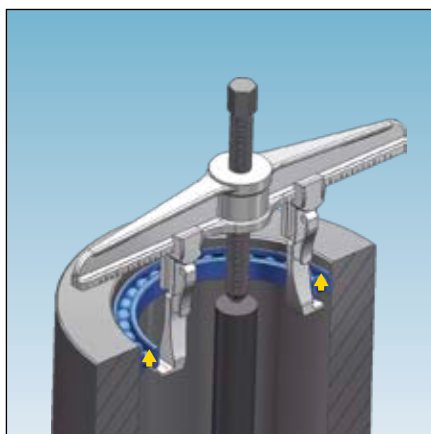
Použití stahováků jednoduchým otáčením stahovacích háků na traverze také jako vnitřní stahovák. Předpokladem je hřídel uprostřed dílu, o který se vřeteno opře.
